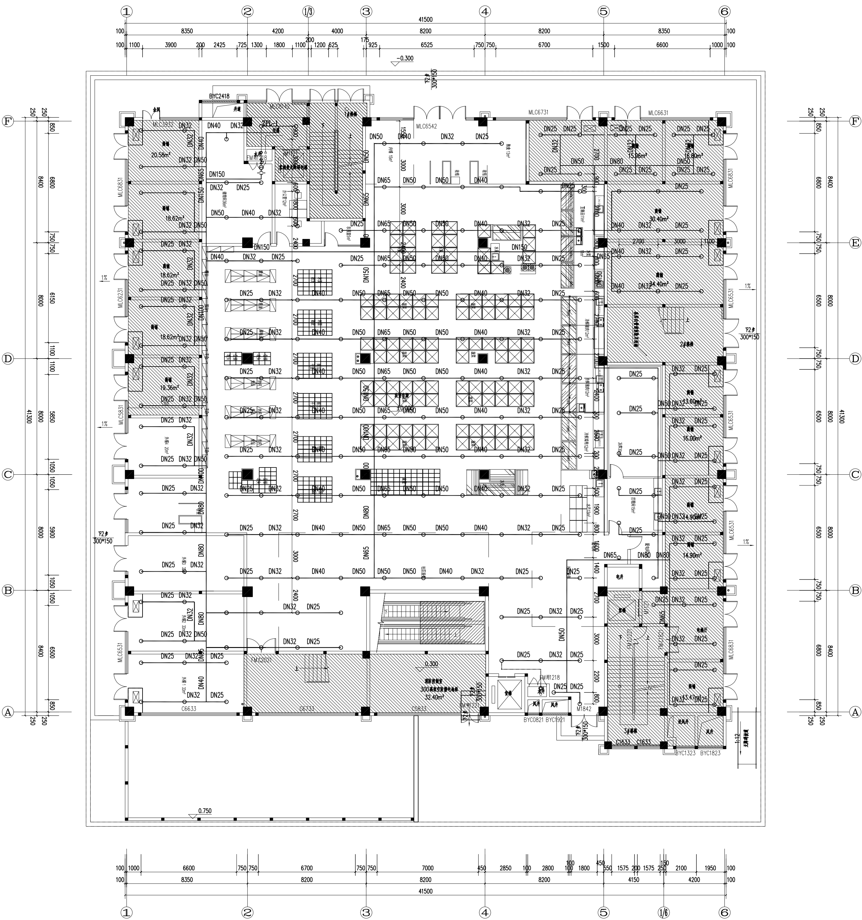
自动喷淋平面图 1:160
